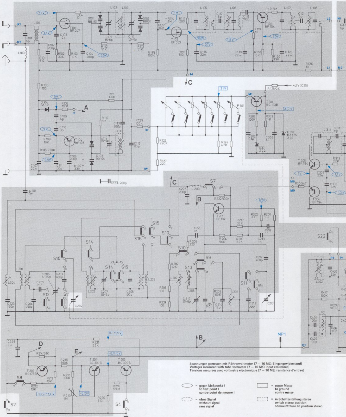
Fig. 2 Schaltbild HF
