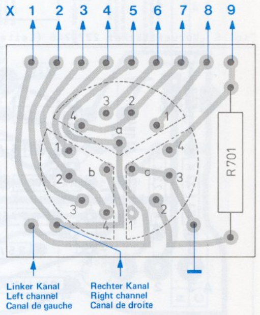
Fig. 8 Betriebsartenschalterplatte 234 473 (Leiterseite)
